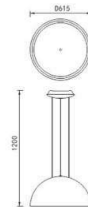
P15006-76W POWER : 76W SIZE(mm) : D615×1200 COLOUR : WHITE
