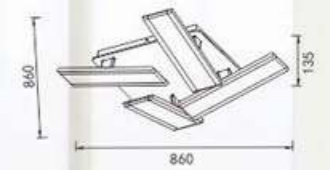
C17600-90W-S POWER : 90W SIZE(mm) : L860×W860×H135 COLOUR : GLOD
