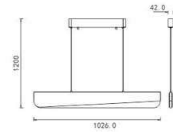
P17803-48W POWER : 48W SIZE(mm) : L1026×W42×H1200 COLOUR : GLOD/GREEN/BLACK
