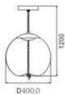
P17813-18W-A POWER : 18W SIZE(mm) : D400×H1200 COLOUR : SMOKE
