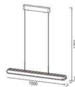
P17001-45W POWER : 45W SIZE(mm) : 1000×72×1200 COLOUR : GLOD
