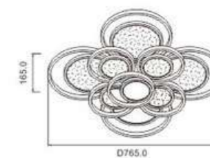
C17808-90W POWER : 90W SIZE(mm) : D765×H165 COLOUR : WHITE//GLOD
