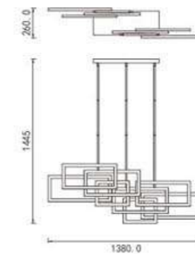
P17801-166W-A POWER : 166.4W SIZE(mm) : L1380×W260×H1445 COLOUR : GLOD
